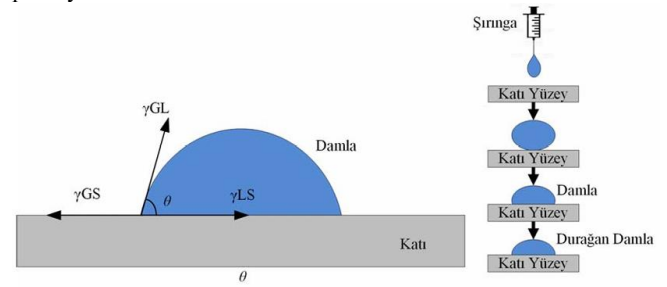
Şekil 4. Yüzey gerilimleri ve statik temas açısı ölçümü sırasında durağan damlamanın oluşumu (Surface tensions. Formation of the sessile drop during static contact angle measurement)
